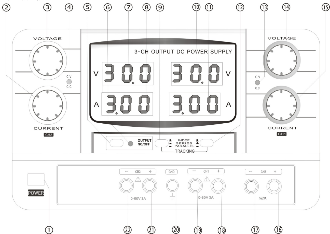
圖 3.1 前面板
