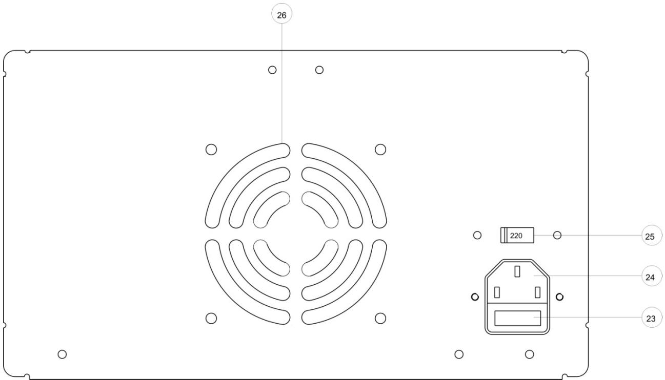
圖 3.2 後面板
